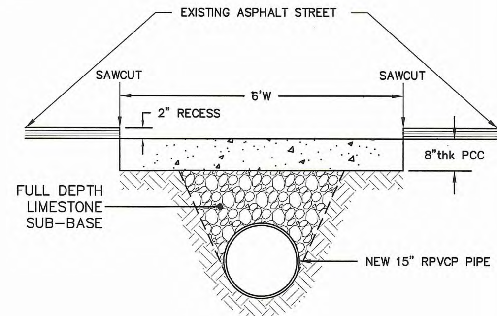
C SECTION A-A SCALE: 1" = 2'
